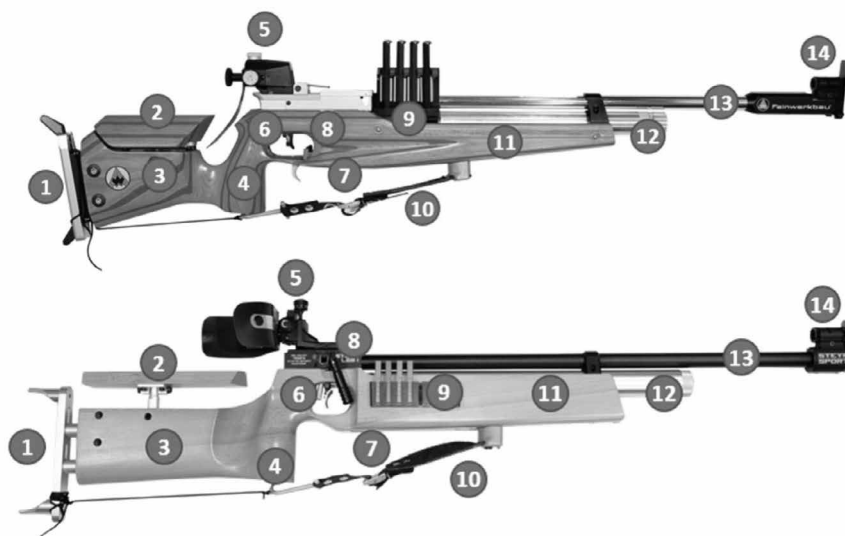
Abbildung 3: Bestandteile eines LG- Biathlongewehrs
