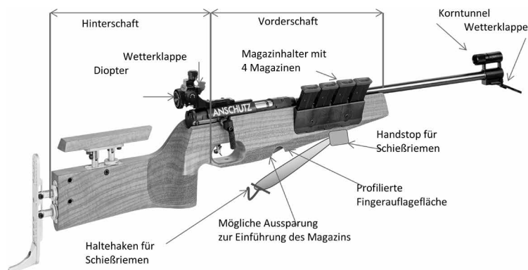
Abbildung 2: Bestandteile eines KK- Biathlongewehrs
