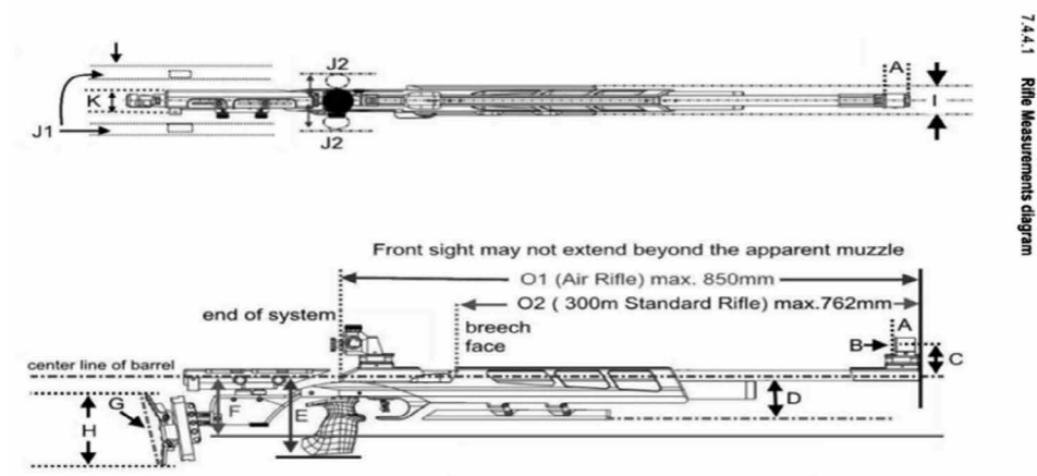
Abbildung 6: Abmessungen des eingesetzten Gewehres
