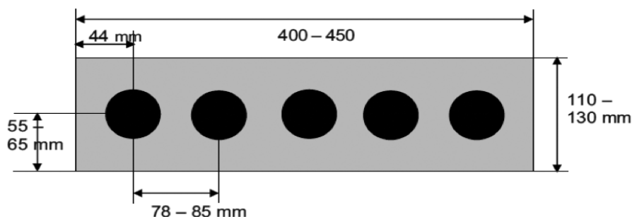
Abbildung 5: Abbildung einer Luftgewehr-Klappscheibe für Target Sprint und Sommerbiathlon
